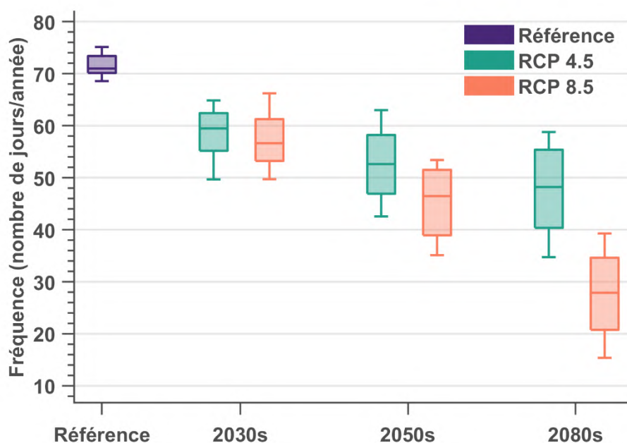
Figure 2.9: Nombre d'événements de gel profond (Temp. min. quotidienne < -10^{\circ}\text{C} )
