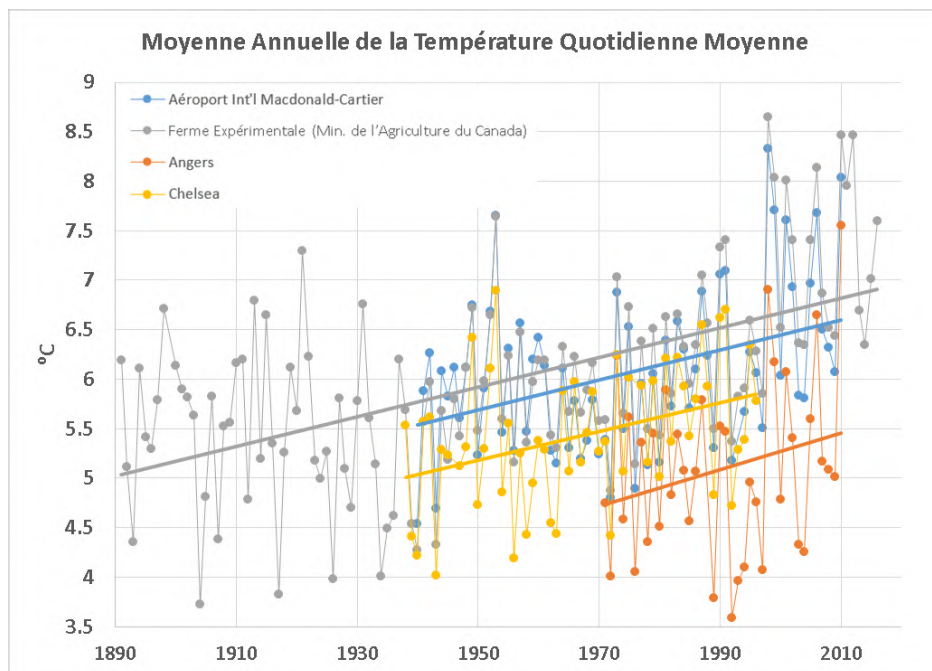
Figure 2.1: Tendances observées de la moyenne annuelle de la température moyenne quotidienne dans la RCN (stations climatiques d'ECCC)
