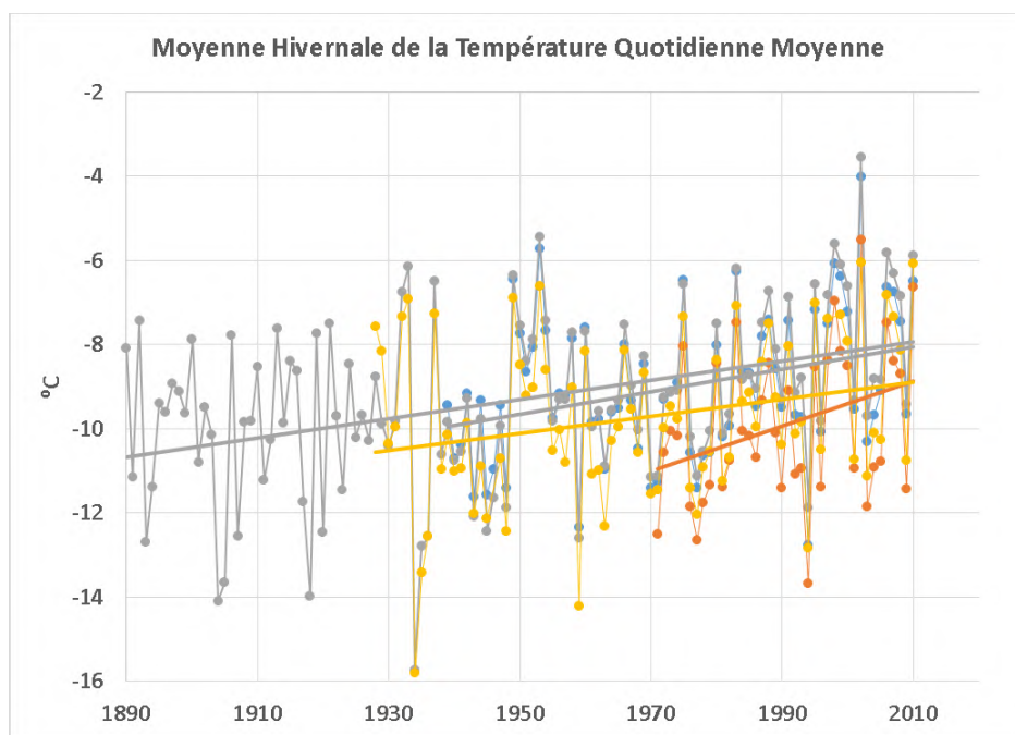
Figure 2.2: Tendances observées de la moyenne de la température hivernale quotidienne dans la RCN (stations climatiques d'ECCC)
