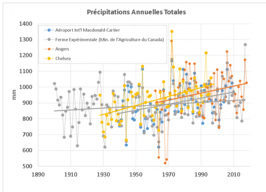
Figure 2.3: Tendances observées des précipitations annuelles totales (stations climatiques d'ECCC)
