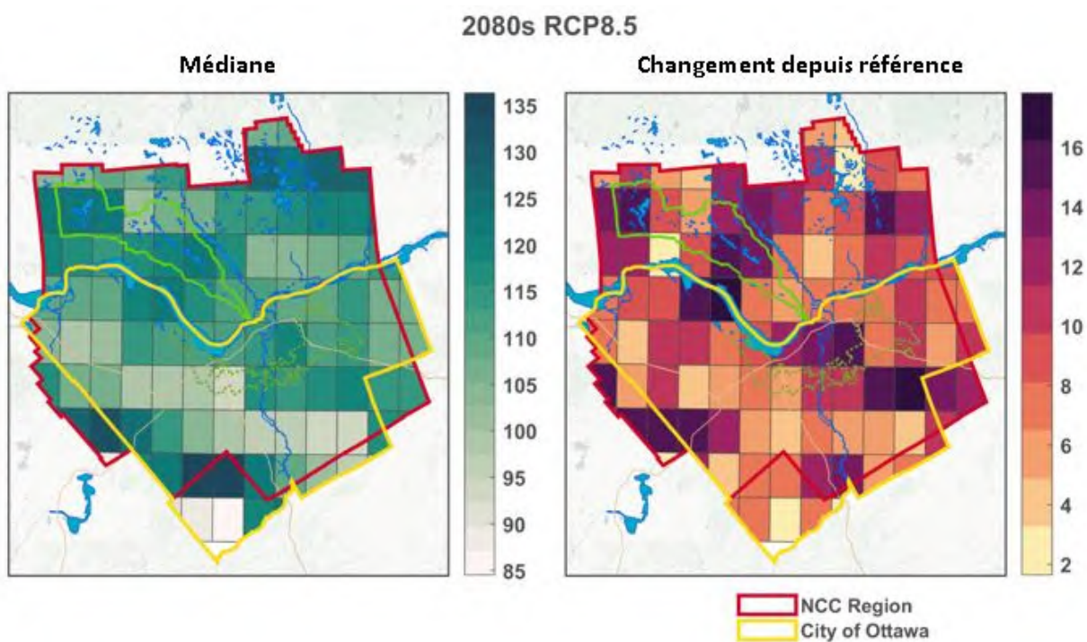
Figure D3 : Exemples de cartes de précipitations extrêmes (événement à récurrence de 100 ans, 24 heures)
